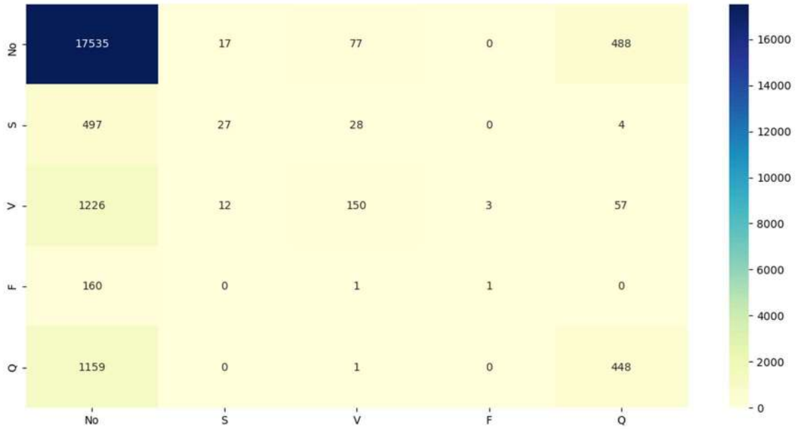
Şekil 3.15. Hata matrisi
