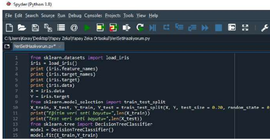
Şekil 1.23. Modeli eğitme
