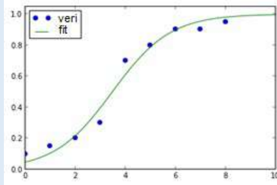
Şekil 1.22. Fit eğrisi
