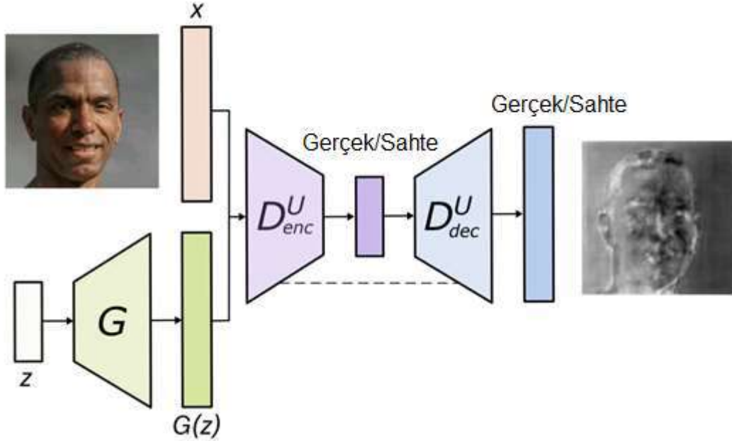
Şekil 8.4. GAN model şeması (Web Kaynağı 8.4)
