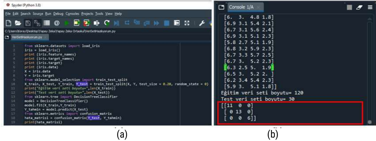
Şekil 1.25. Hata matrisi a) kod b) sonuç görüntüsü
