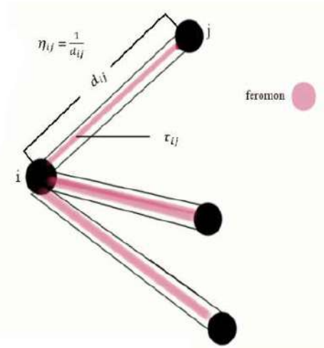
Şekil 7.5. Karınca Koloni Optimizasyonu içerisinde atılacak yeni adımların hesaplanması
