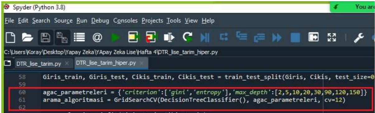
Şekil 4.17. Karar ağacı hiper parametrelerin tanımı ve GridSearchCV algoritmasının uygulanması
