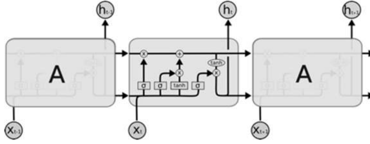
Şekil 8.6. LSTM Network Yapısı (Web Kaynağı 8.5)
