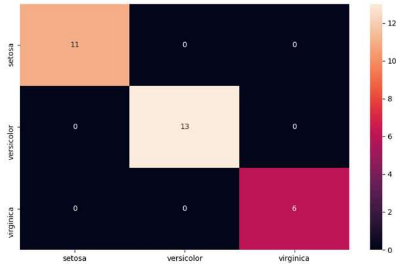
Şekil 1.26. Hata matrisi
