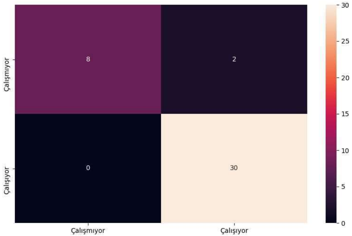
Şekil 5.13. Hata matrisi
