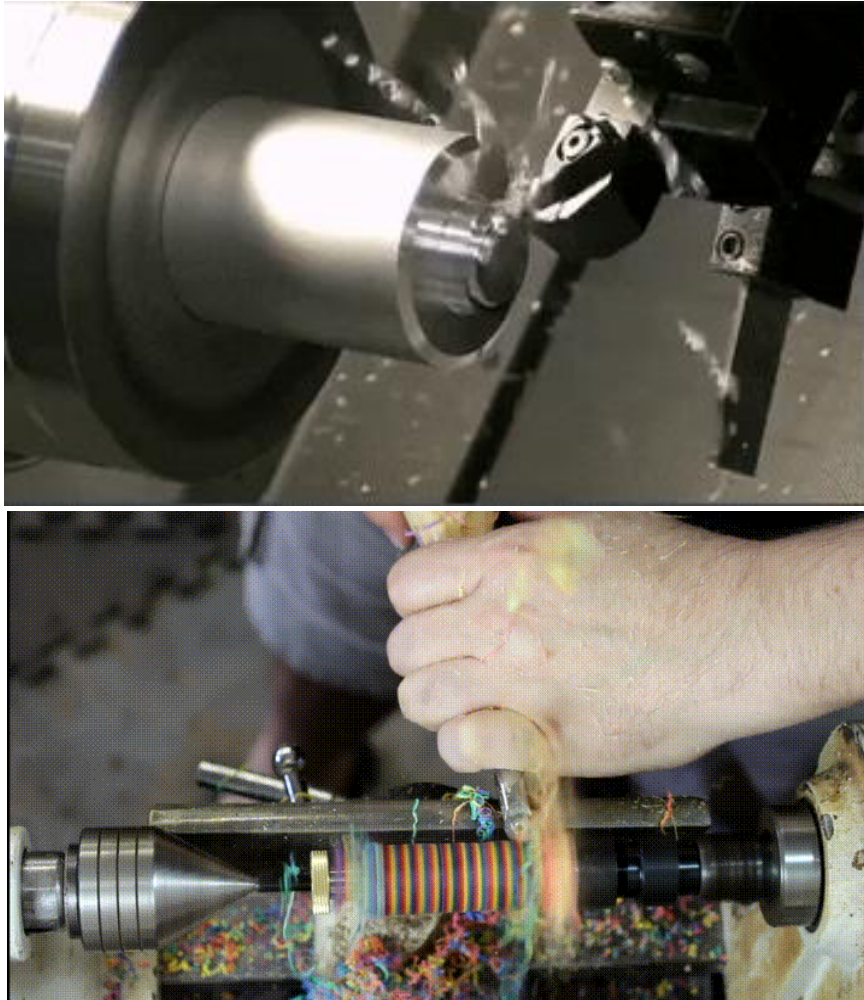
Şekil 1.6. Tornalama çalışma prensibi (kaynak: üst: https://giphy.com/shockingsoggygreathornedowl-cnc , alt: https://giphy.com/gifs/rainbow-wood-lathe-fff1xa9KrY4DK )
